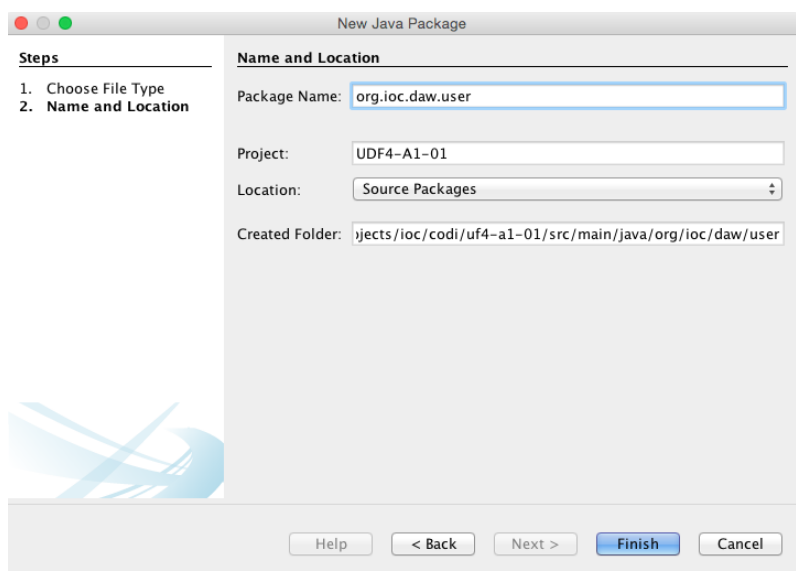
FIGURA 1.18. Paquet org.ioc.daw
