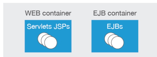
FIGURA 2.4. Contenidor d'EJB
