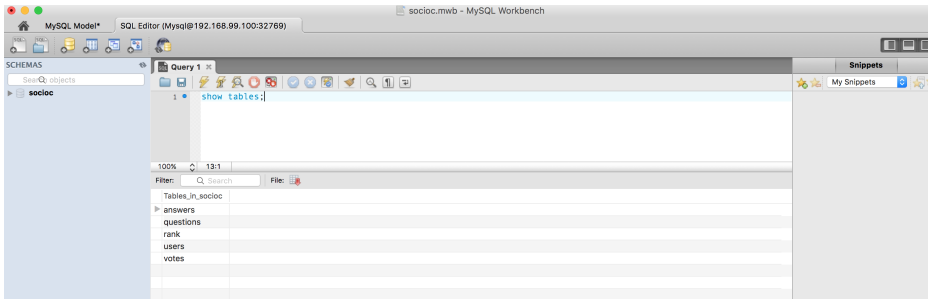
FIGURA 2.10. Editor SQL
