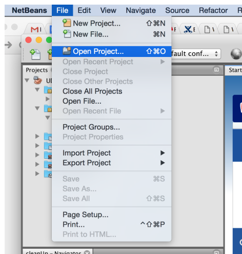
FIGURA 2.11. Editor SQL
