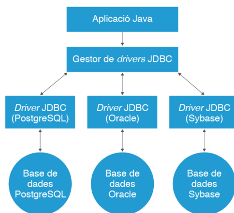
FIGURA 1.4. Arquitectura JDBC
