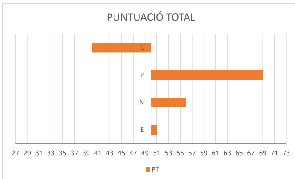
Fig. 5-Representació gràfica de les puntuacions T obtingudes per un subjecte en el qüestionari EPQ-R.
